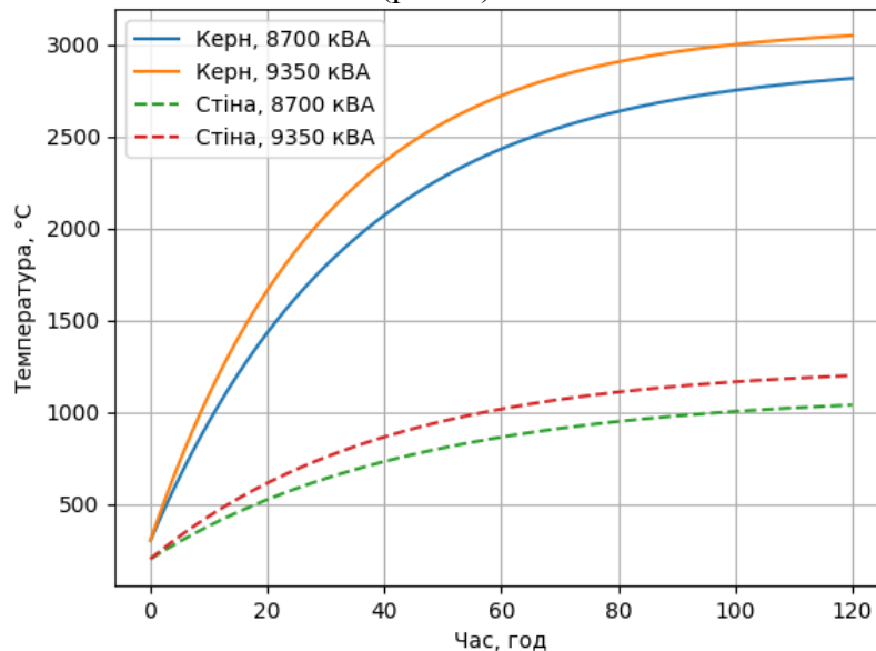
Рисунок 1 – Динаміка температури на керні і стінках печі Ачесона під час процесу графітації
