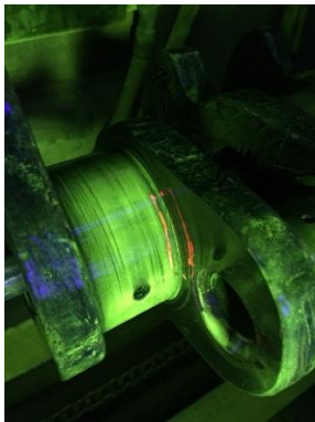
Рисунок 2 – Магнітнопорошковий метод вимірювання
