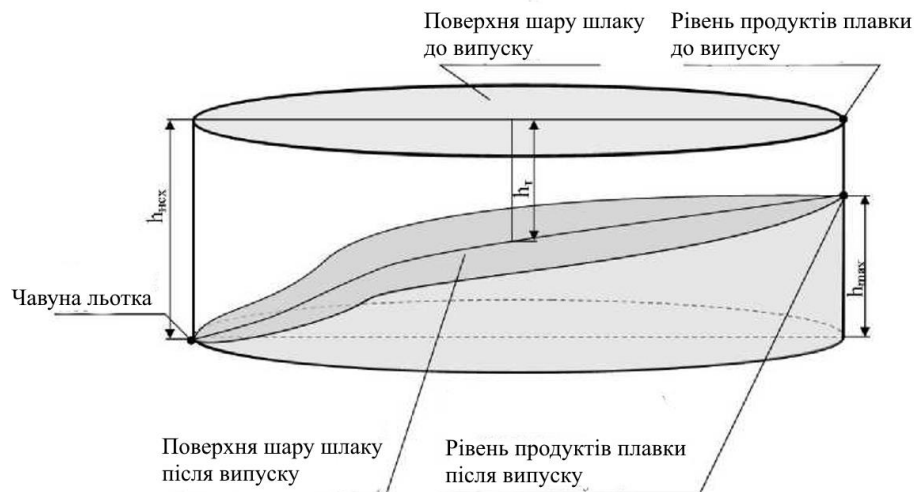
Рис. 1 - Схема розташування шарів шлаку і чавуну в горні доменної печі до і після випуску чавунка
