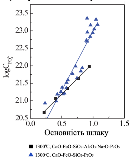
Рис. 1 - Залежність фосфатної ємкості шлаку від основності
