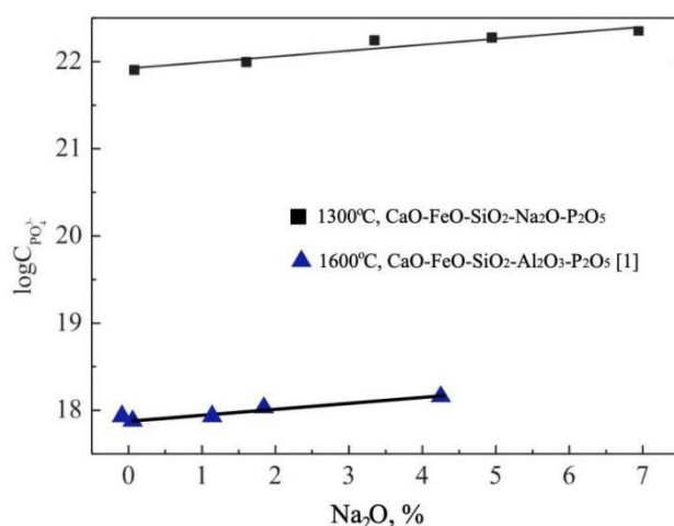
Рис. 2 - Вплив Na 2 O на фосфатну ємкість шлаку в залежності від температури
