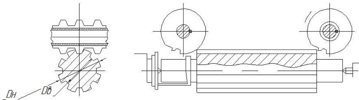
Рисунок 2 – Схема фрезерування шліців на валу черв'ячною фрезою
