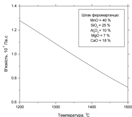
Вплив температури на в'язкість феромарганцевого шлаку
