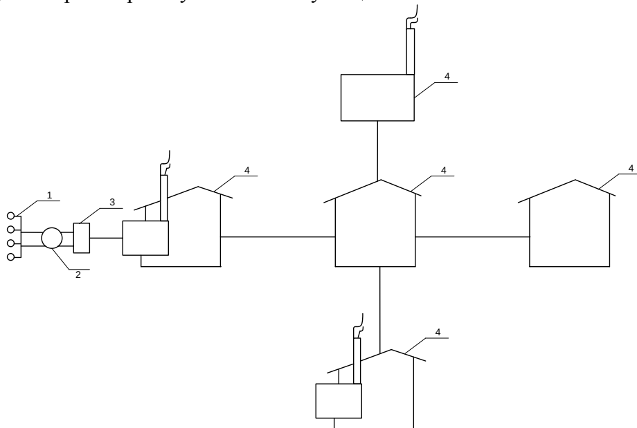
Рис.1. Схема районної системи водопостачання
